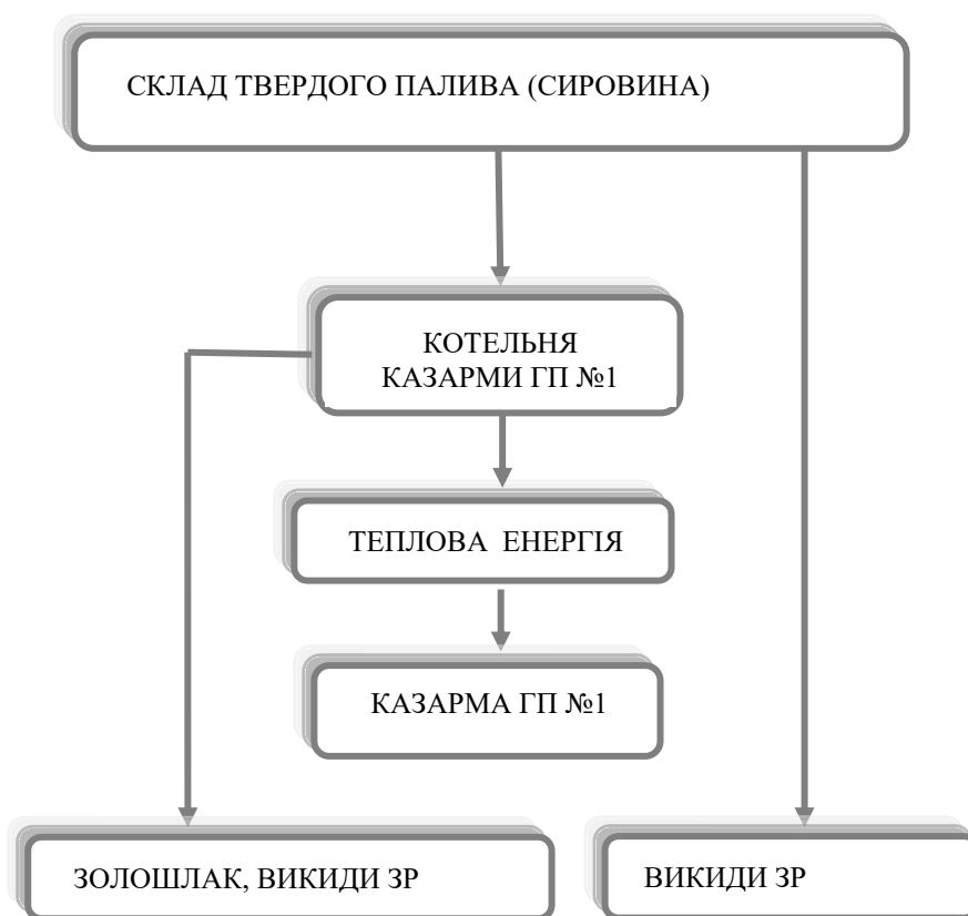
Мал.3 Блок-схема виробничого процесу на проммайданчику в/м №Дальник-7
